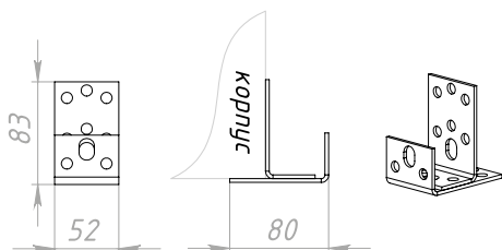
Topvex FR03
