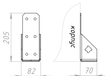
Topvex FR06-11
