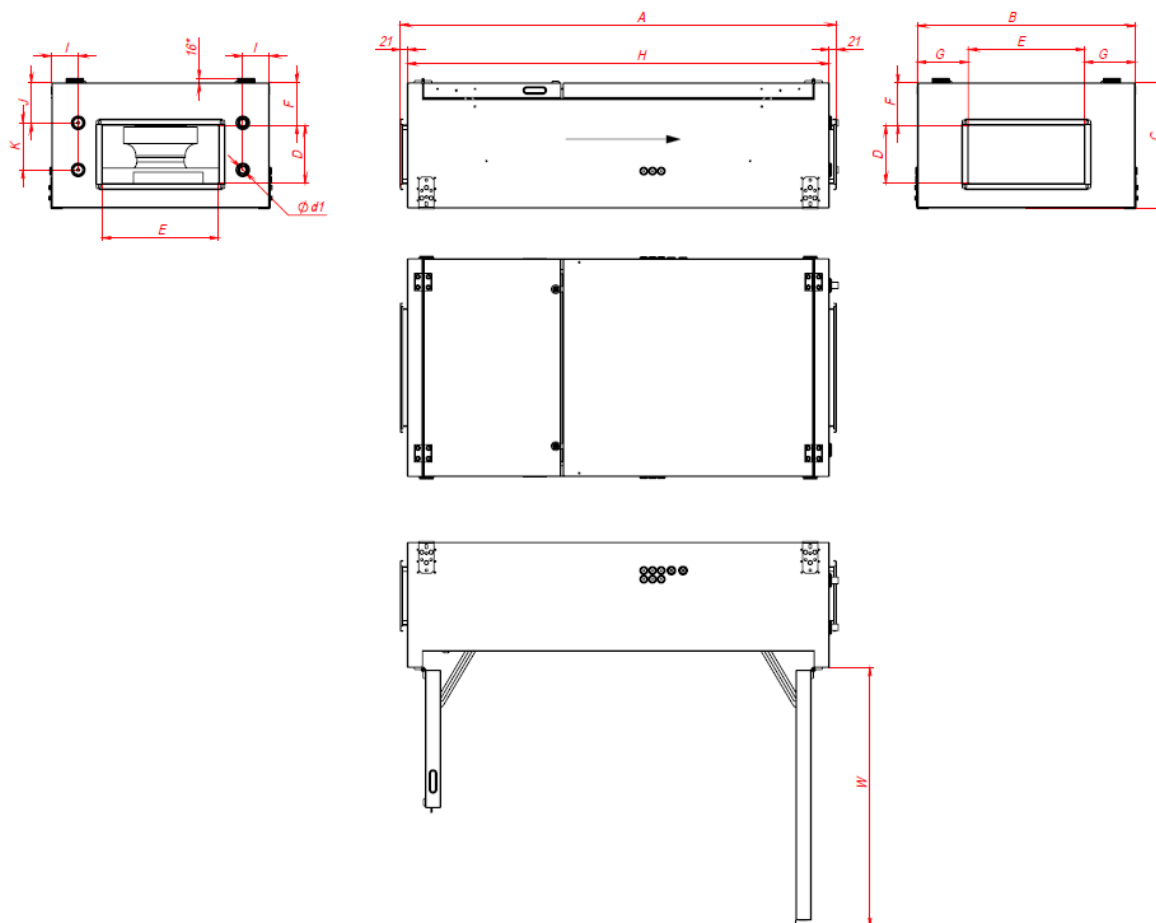
Рис.2 Габариты и присоединительные размеры Topvex SF04, SF08 и SF12
