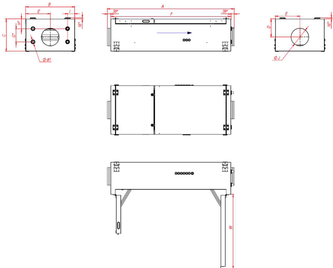
Рис.1а Габариты и присоединительные размеры Torvex SF02
