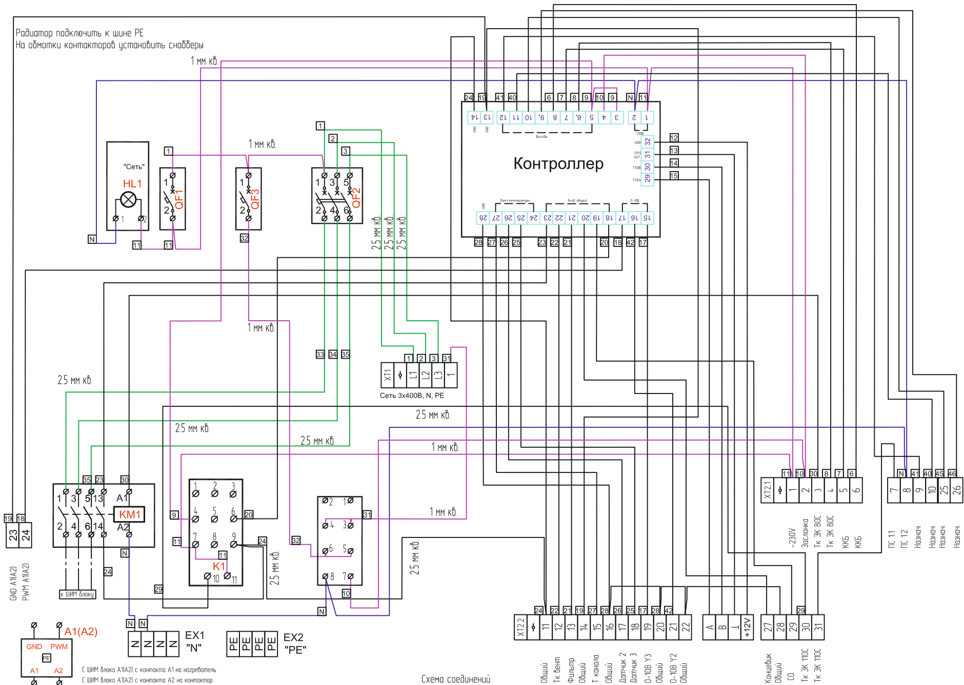
Схема соединений Проводники, для которых сечение не указано выполнить проводом сечением 0,5 мм кв.
