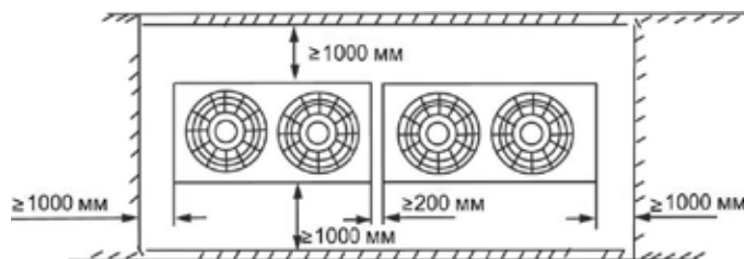
Вид агрегатов сверху (схема монтажа нескольких агрегатов)
