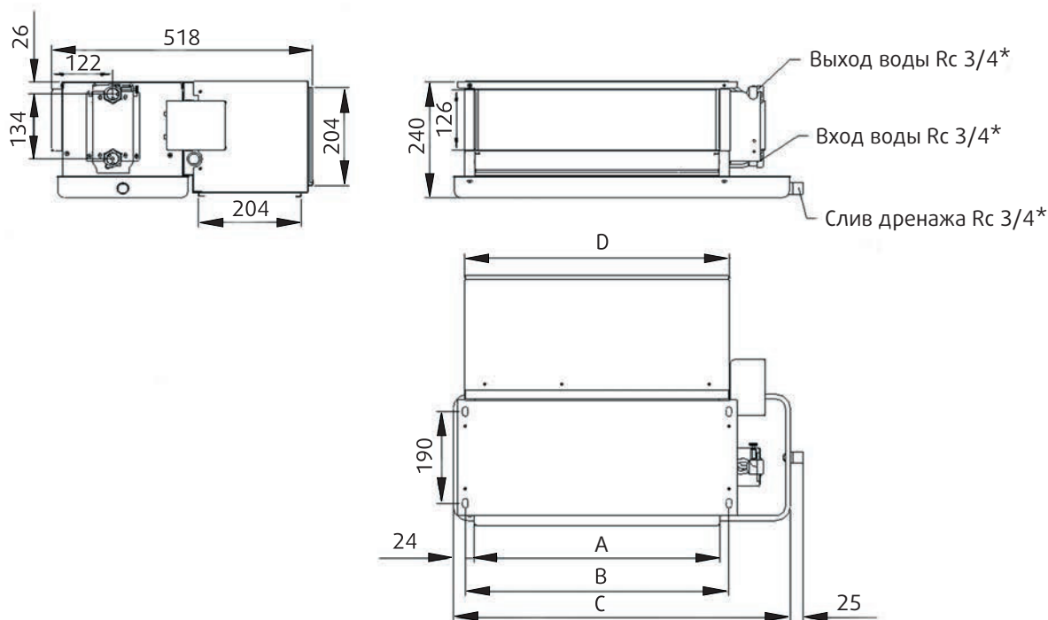
Габариты, мм
