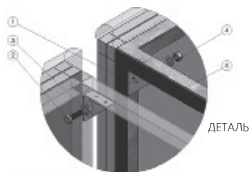
ДЕТАЛЬ А
