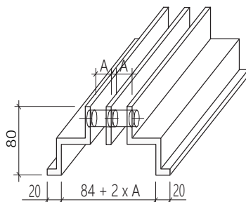
исполнение 2
