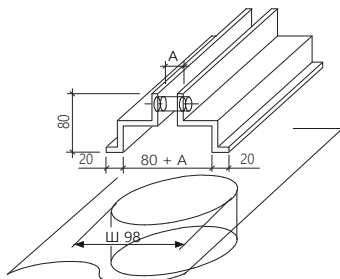
исполнение 1
