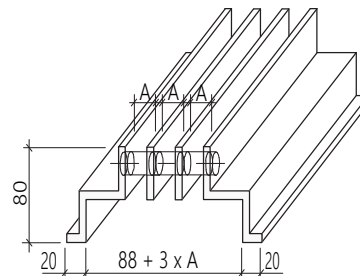
исполнение 3
