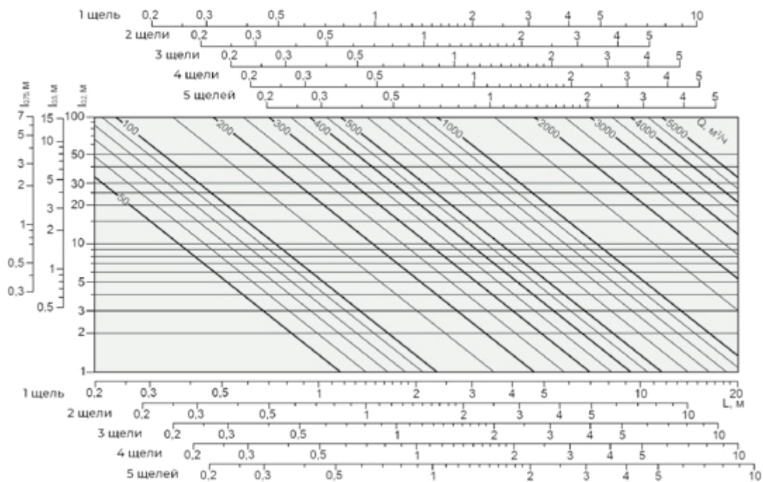
Горизонтальное направление струи (схема 2)
