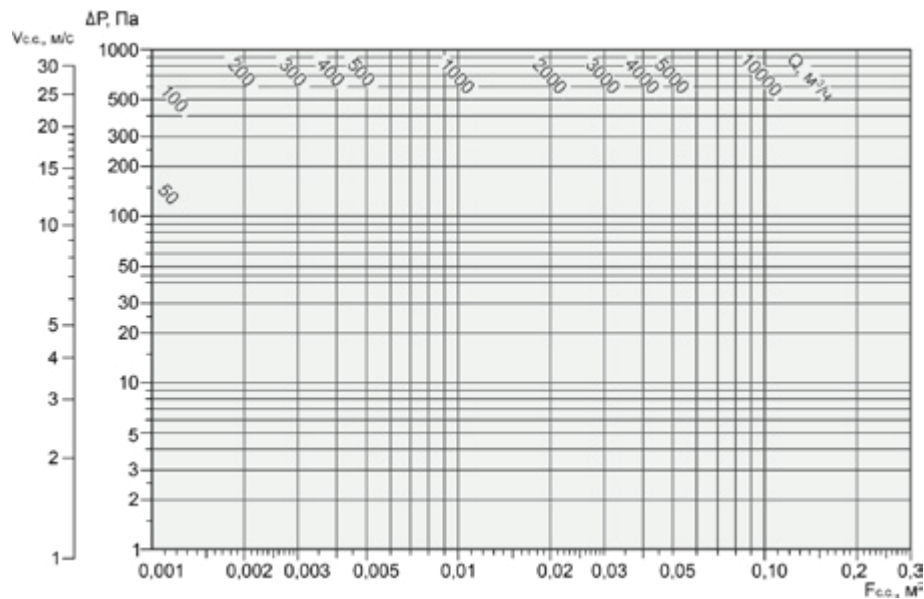
Горизонтальное направление струи (схема 2)
